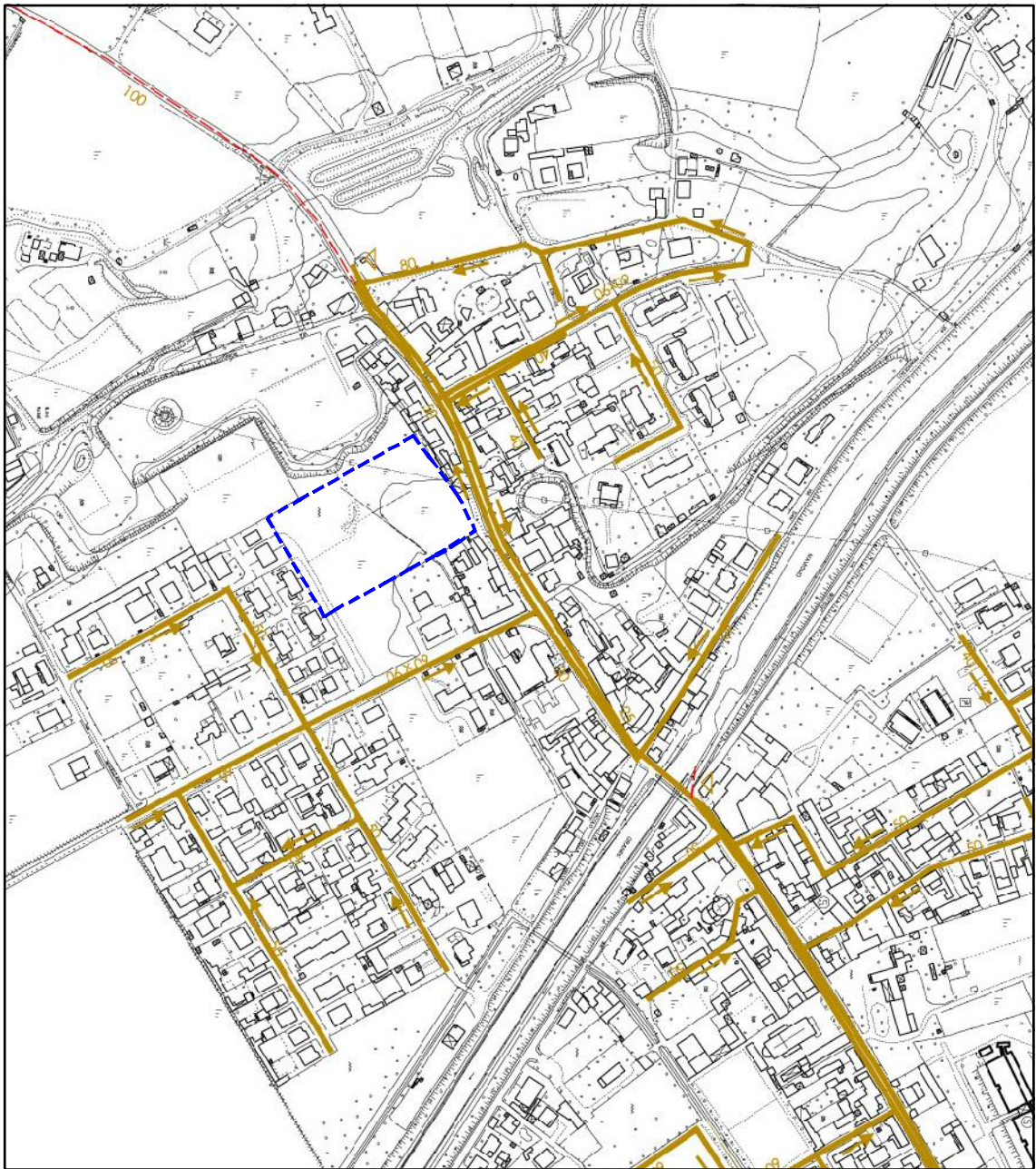
SCHEMA RETE PUBBLICHE FOGNATURE
